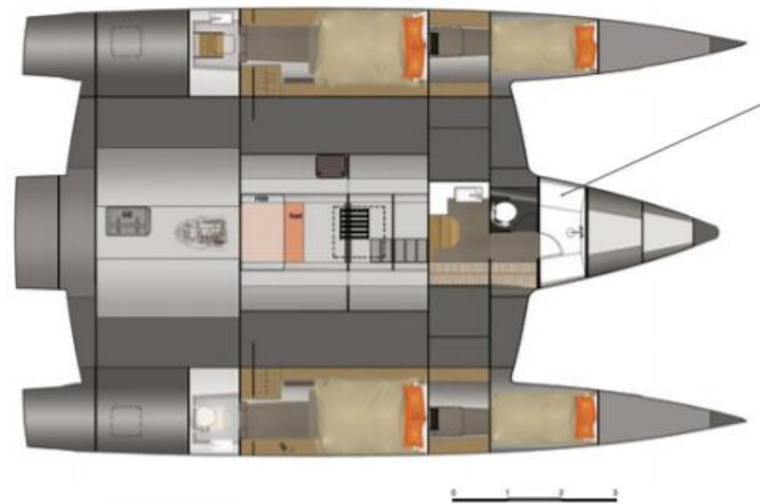
Coque centrale et flotteurs
